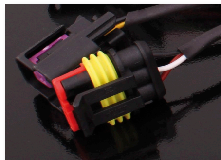
Fig 4.1a - 3-poliga Superseal kontakt.
